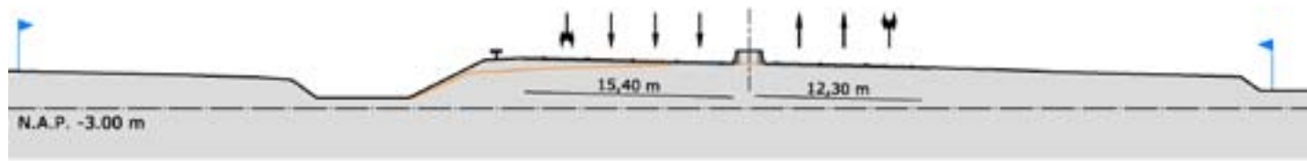
profiel nieuwe situatie (in oranje bestaand maaiveld)
