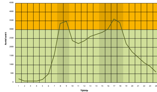
— Hoeveelheid verkeer die de zuidelijke ringweg tijdens de bouwwerkzaamheden kan verwerken bij het gebruik van 2 x 2 rijstroken — Verkeersintensiteit gedurende een etmaal
