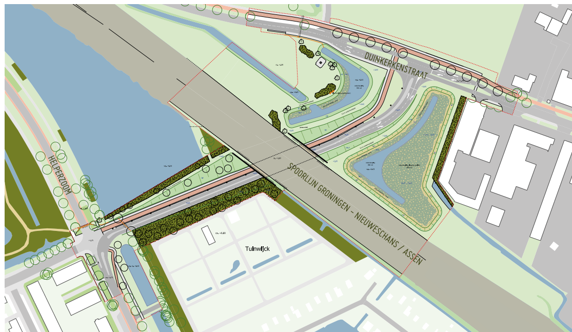
Ontwerptekening Helperzoomtunnel (aansluiting fietsverbinding Helperzoom in ontwikkeling)
