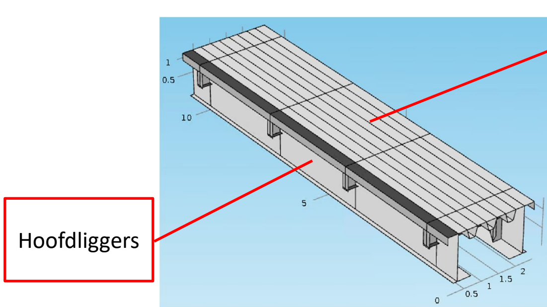
Figuur 3 – Model RHB element
