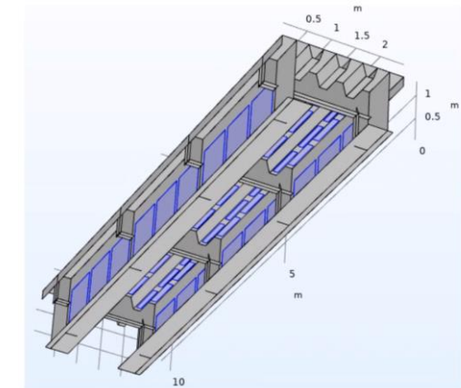
Figuur 6 – CLD-panels op het element
