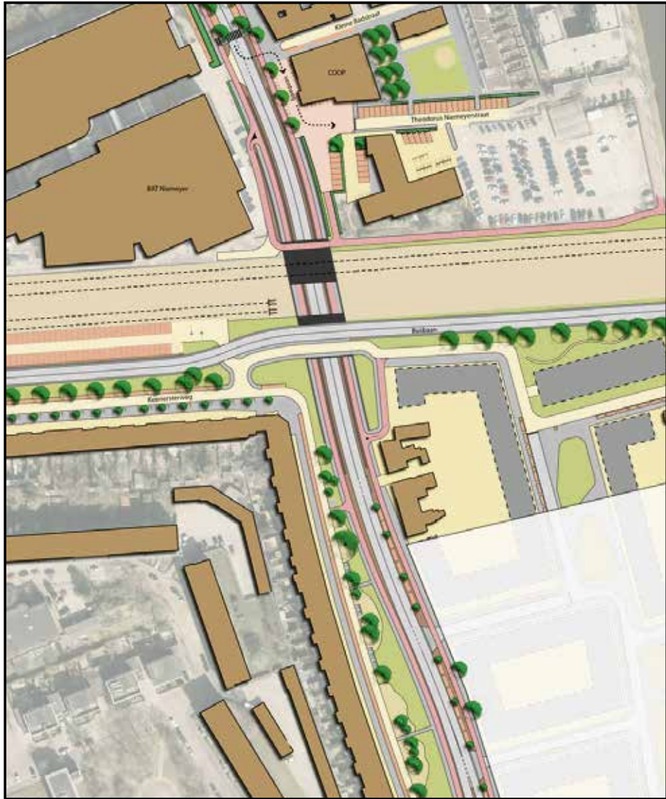
SCHETS VAN DE NIEUWE SITUATIE BIJ DE PATERSWOLDSEWEG. DE STIPPELIJN IS HET SPOOR TUSSEN GRONINGEN EN LEEUWARDEN. DE PATERSWOLDSEWEG GAAT HIER ONDERDOOR. DE VERLENDE BUSBAAN LIGT AAN DE ZUIDKANT VAN HET SPOOR. BRON: GEMEENTE GRONINGEN
